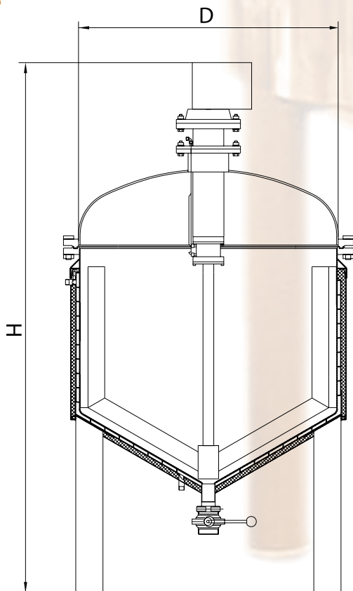
цялостно изпълнение от AISI 316 целостное выполнение из AISI 316 performance from AISI 316
